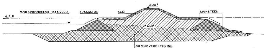
DOORSNEDE A-A
