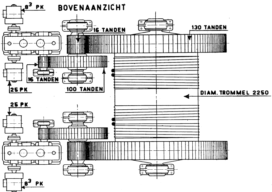
Bewegingswerk voor de schuif
