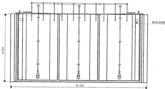
EENHEIDSCAISSON
