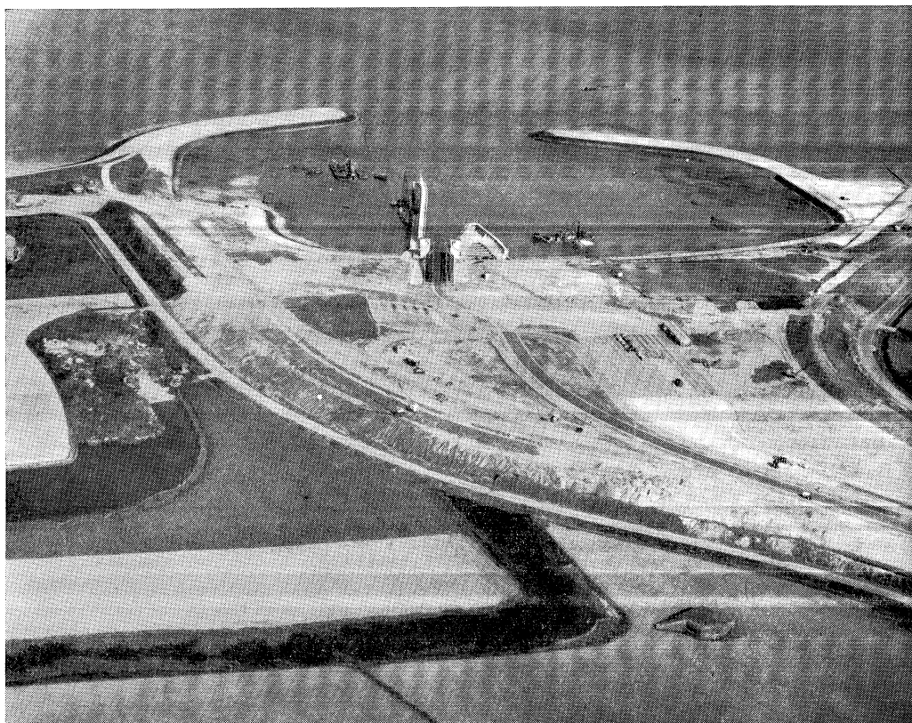
De nieuwe veerhaven te Breskens tijdens het afwerken van de waterkering
