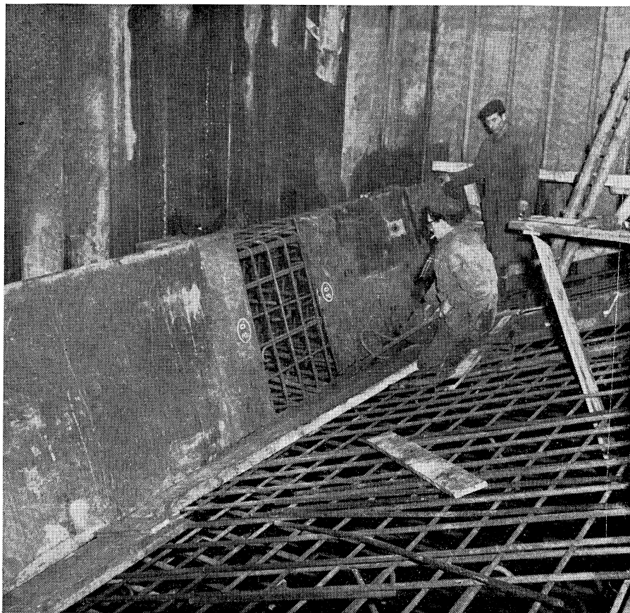
De betonnen drempel waarop de schuif komt te rusten in aanbouw
