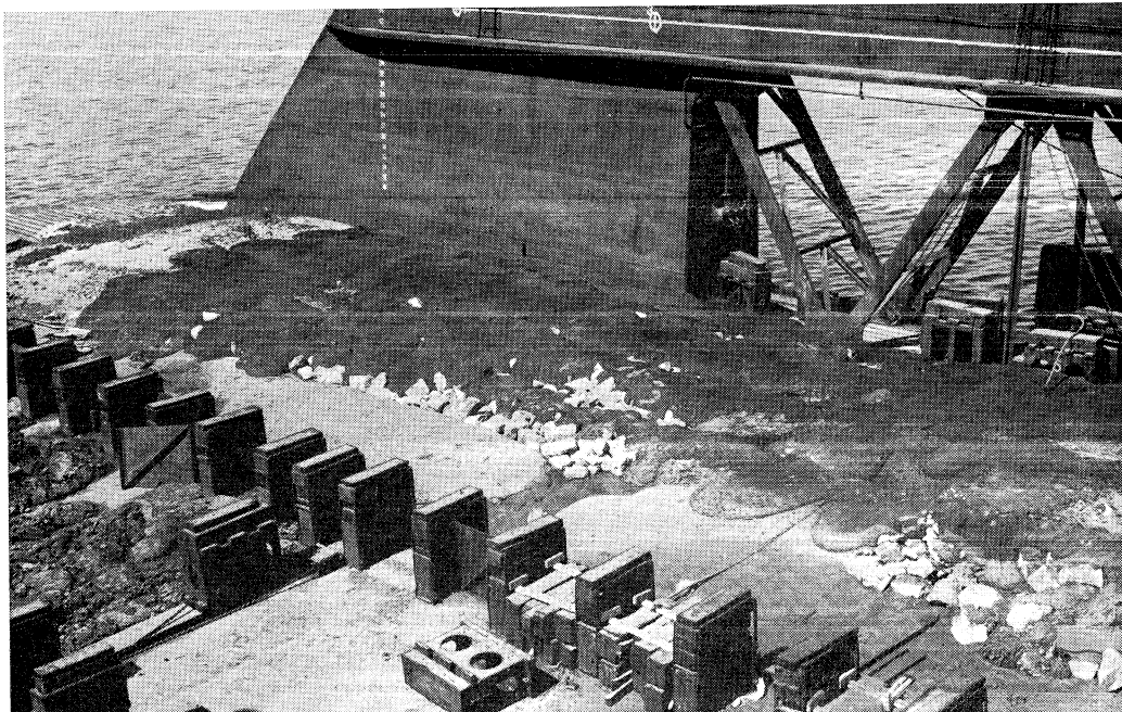
Het proefvak in het dok na het storten met vier stralen
