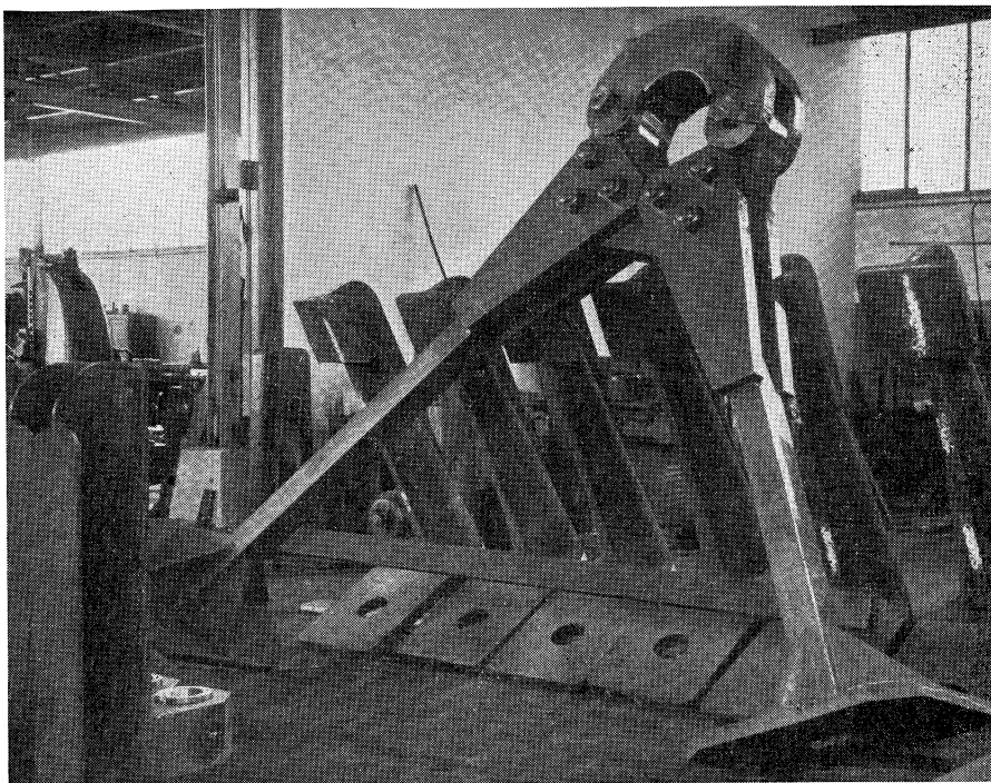
Halsbeugel
