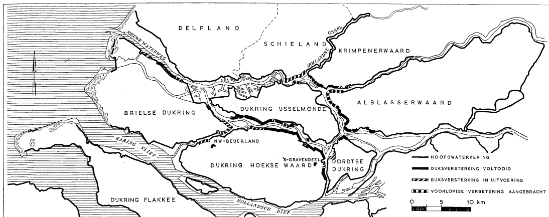
Stand van de versterking der bestaande hoogwaterkeringen in het Deltagebied op 1 oktober 1957
