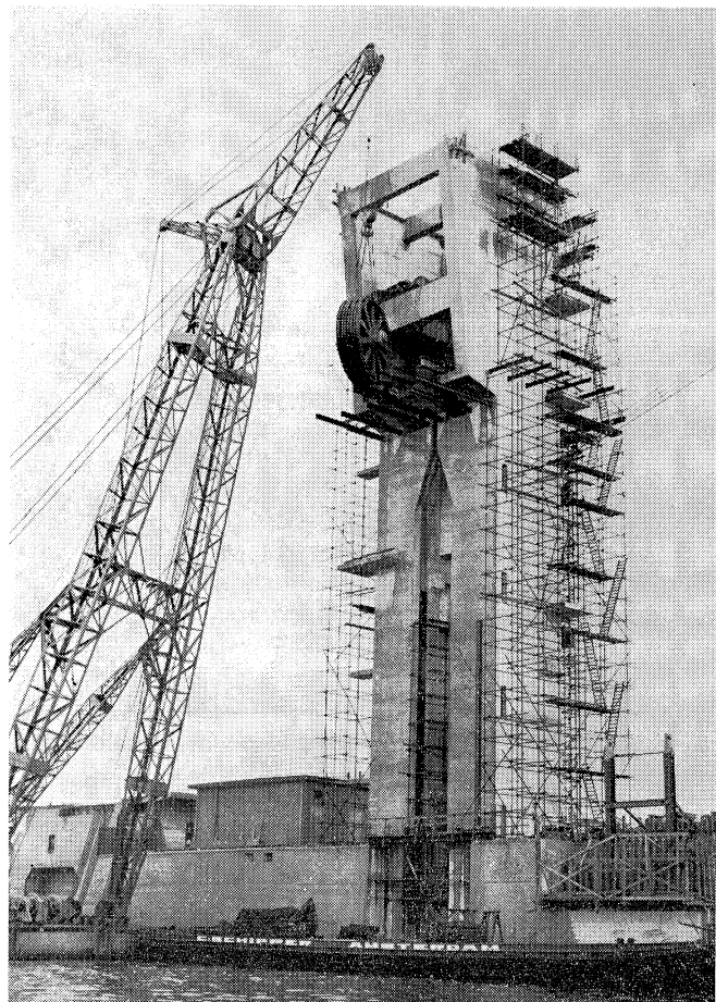
Montage van de kabelwielen
