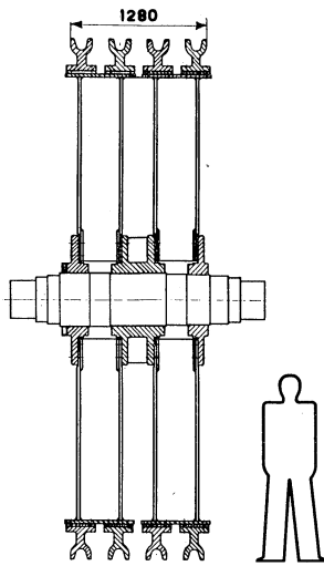
DOORSNEDE
