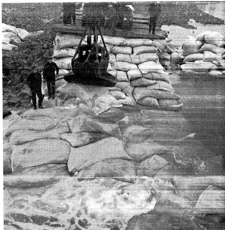
In het sluitgat is de stroom gebroken
