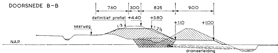
DOORSNEDE B-B
