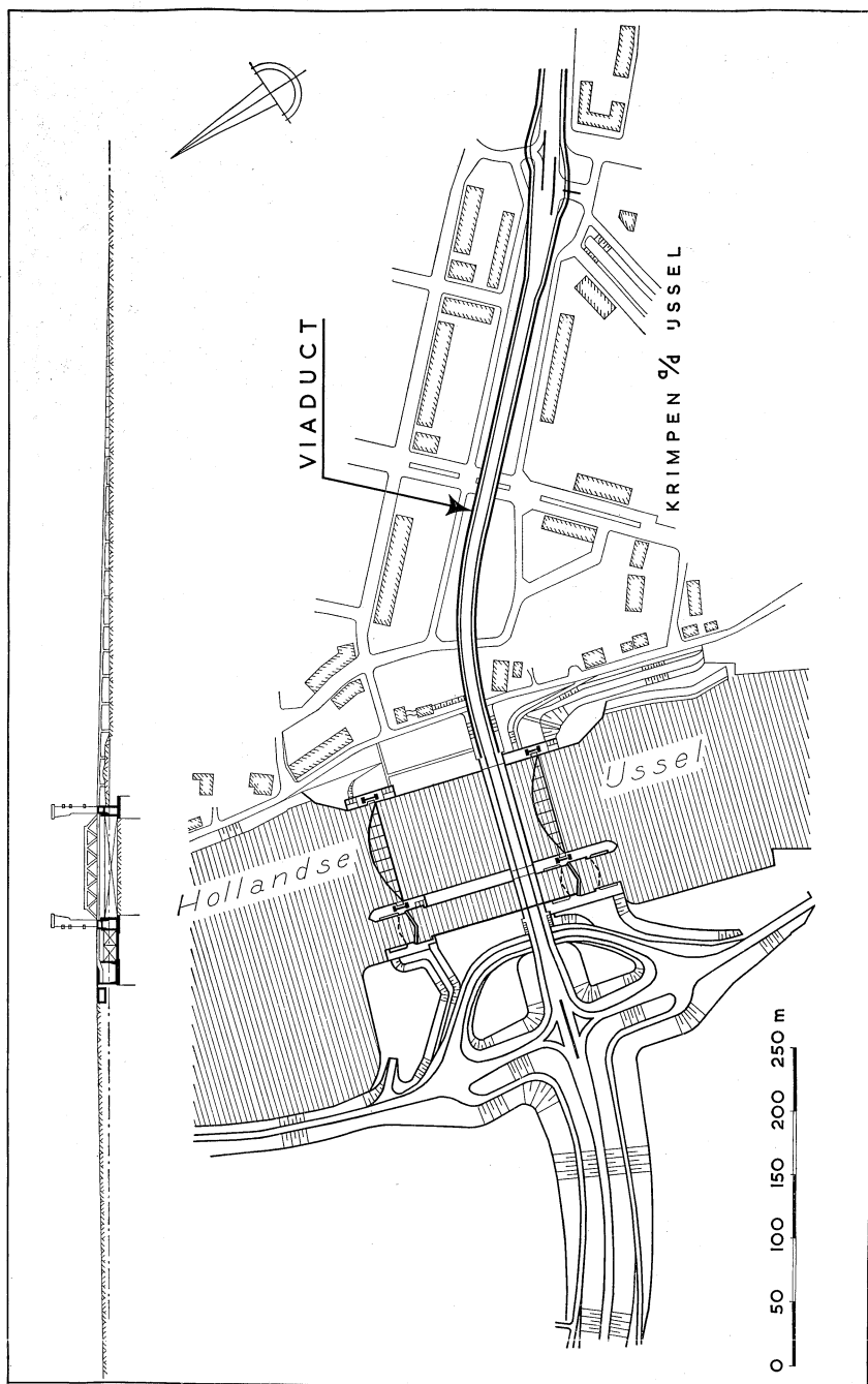
Situatie en langsdoorsnede van de wegverbinding
