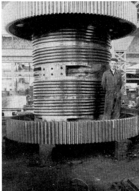
Kabeltrommel voor bewegingswerk van de schuif
