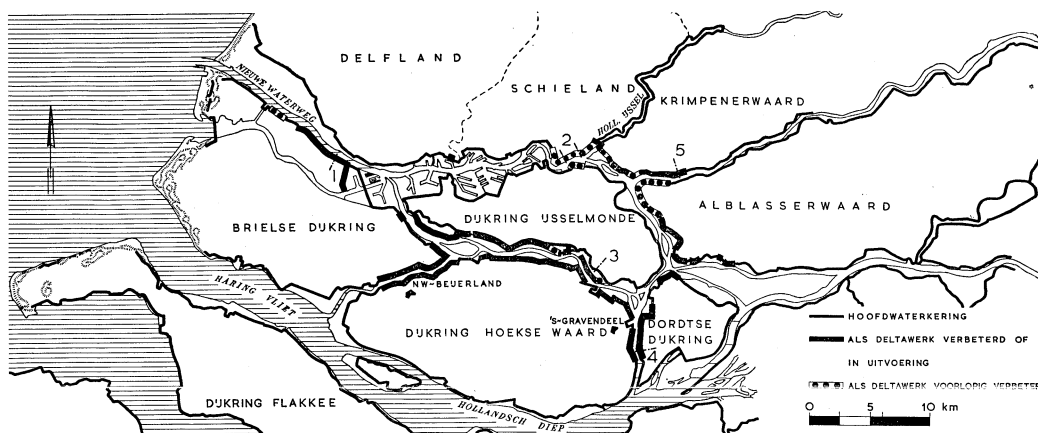
Stand van de versterking der bestaande hoofdwaterkeringen in het Deltagebied op 1 juli 1958
