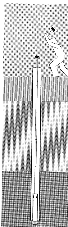
Steekapparaat
