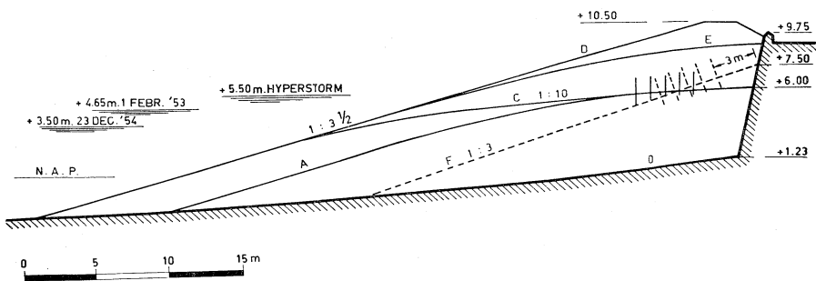
Profielen van diverse bermtypen, beproefd in de windgoot van het Waterloopkundig Laboratorium te Delft
