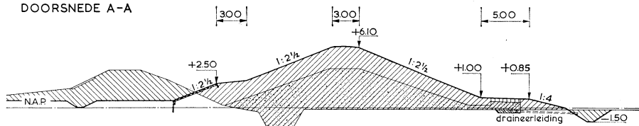
DOORSNEDE A-A
