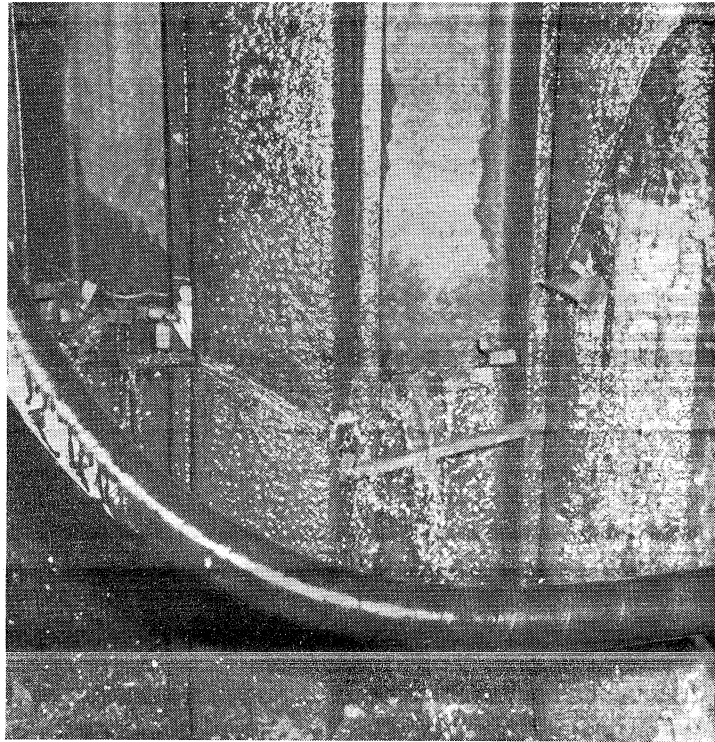
Scheuren in de damwand ter plaatsse van de drempel
