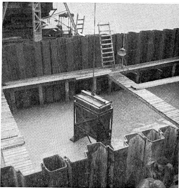
Het storten van beton onder water voor het maken van de drempels. Op de voorgrond zijn de stalen funderingspalen van Larssen-damwand zichtbaar.
