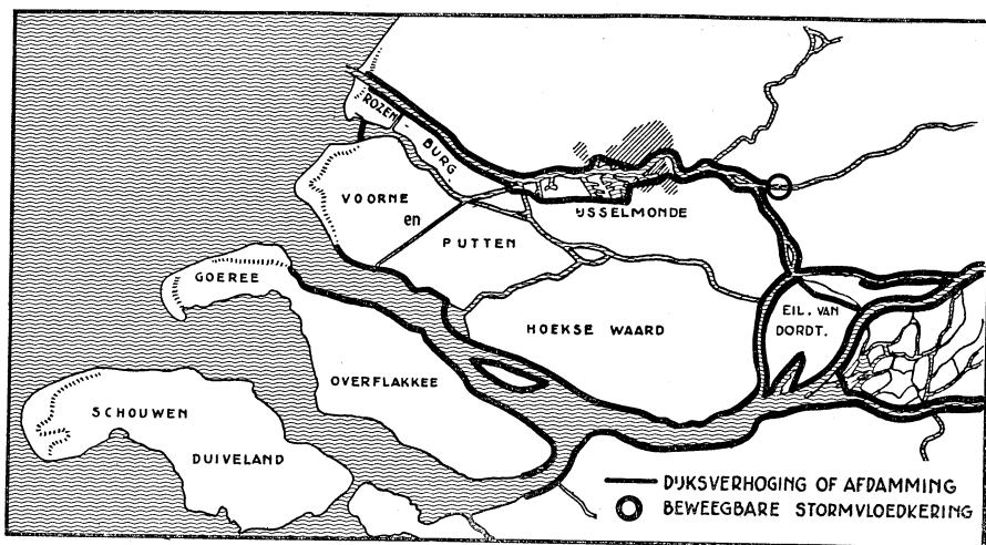
Vier-eilandenplan
