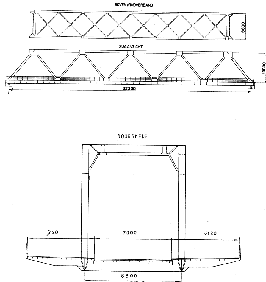
Hoofdafmetingen van de vaste brug
