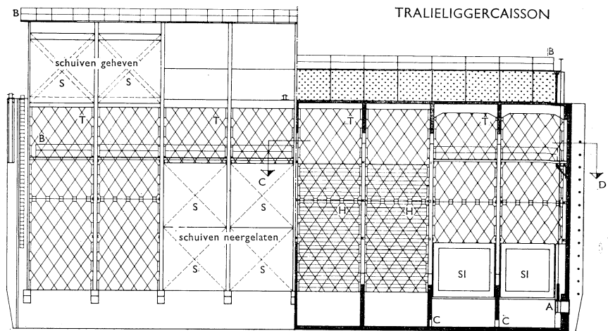
AANZICHT
