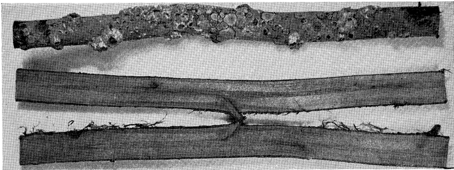
Rijshout behandeld met koper-naftenaat, na één seizoen in zeewater, onaangetast
